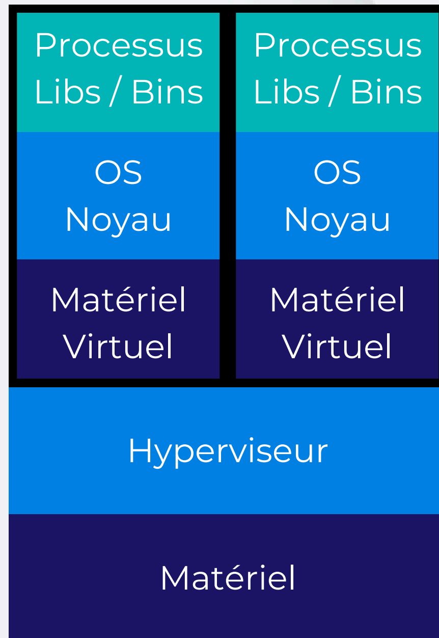
Virtualisation
