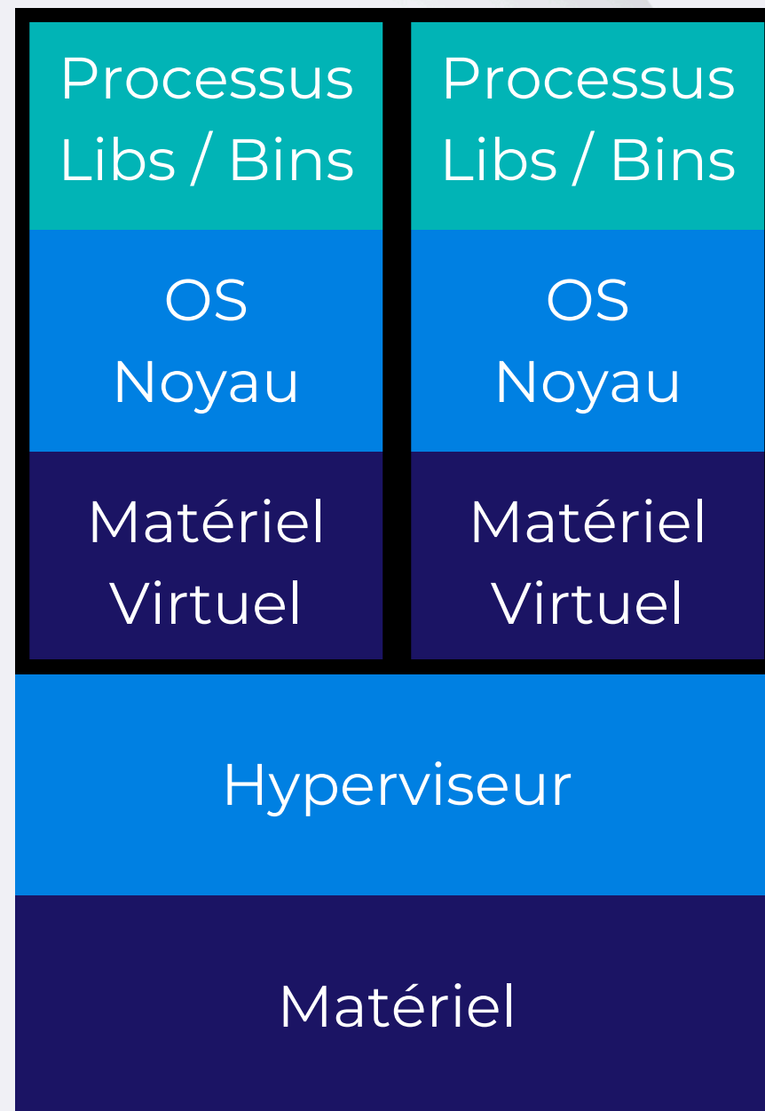
Machine virtuelle
